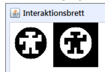
Abbildung 4: robbi()
